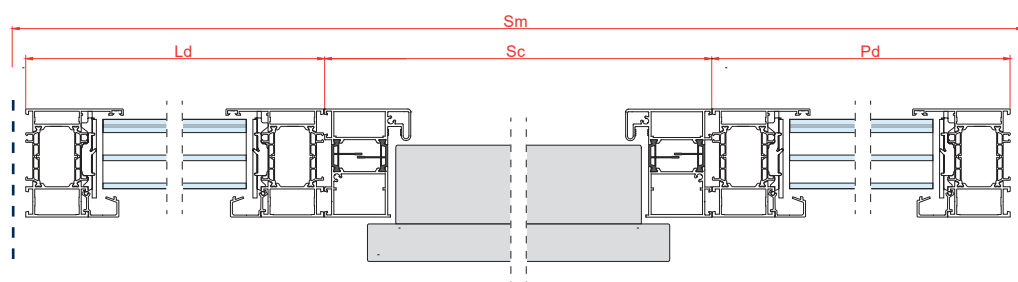
DOŚWIETLA BOCZNE PRZEKRÓJ POZIOMY
