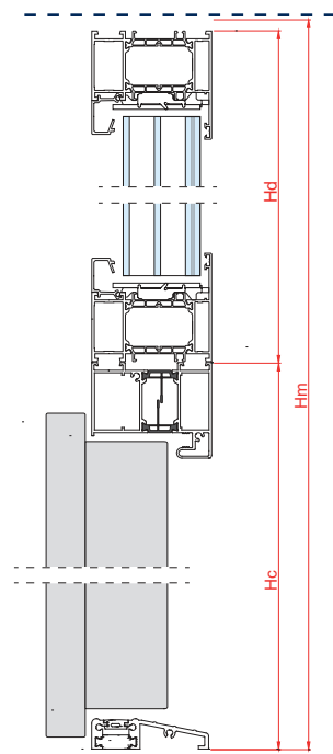
DOŚWIETLE GÓRNE PRZEKRÓJ PIONOWY
