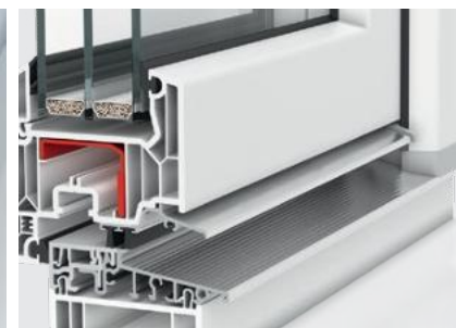
Niski próg aluminiowy
